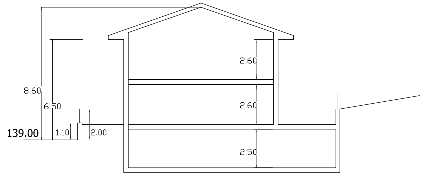
ZEHAR EBAKIDURA 1/250 SECCION TRANSVERSAL 1/250
